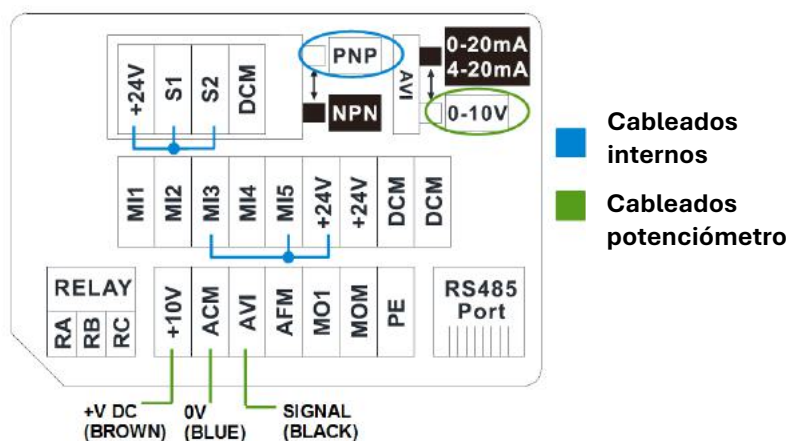
FIGURA 5: control manual - conexión PNP - potenciómetro externo
