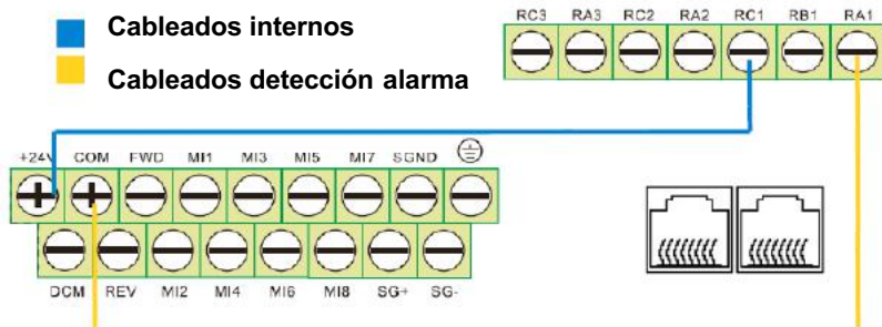
FIGURA 22: Cableados para detección de alarma vía relé
