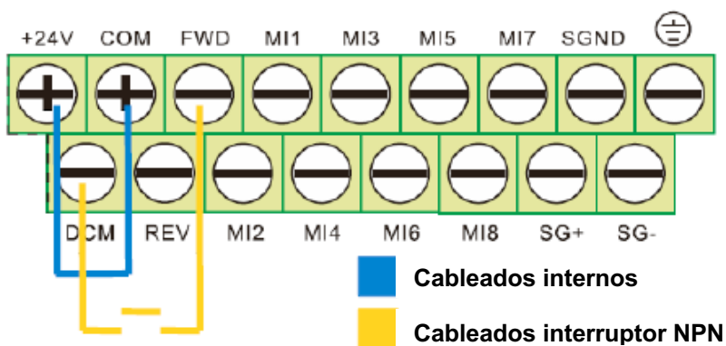
FIGURA 10: operación de interruptor automático/PLC – conexión NPN
